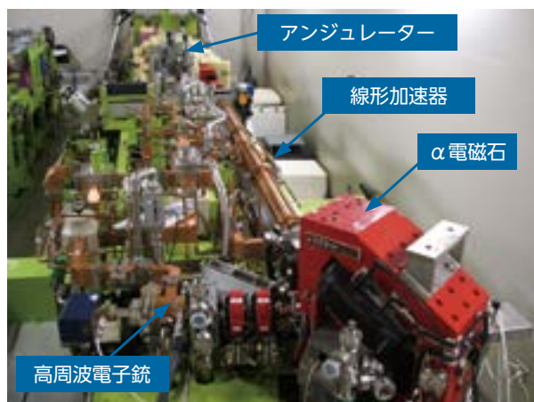
図 1 赤外自由電子レーザー本体
