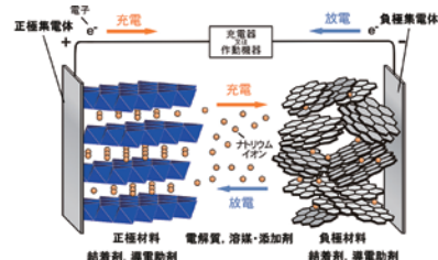
図2 ナトリウムイオン二次電池の構成
