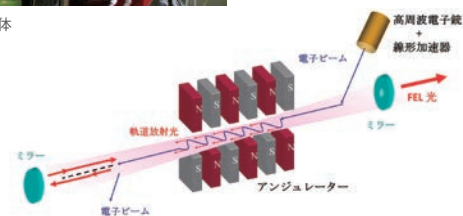
図2 アンジュレーターの構造
