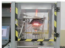
コーンカロリメータ試験装置 (ISO5600)
