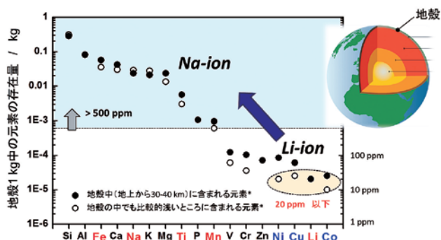
図1 地殻中の各元素の存在量(青字の元素はリチウムイオンで使われている元素、赤字はナトリウムイオンでの活用が期待できる元素を示す) データの典拠: *R.S. Carmichael (Editor), CRC Practical Handbook of Physical Properties of Rocks and Minerals, CRC Press, Boca Raton (1989) **S.R. Taylor, S.M. McLennan, The continental crust: Its composition and evolution, Blackwell Sci. Publ., Oxford (1985)
