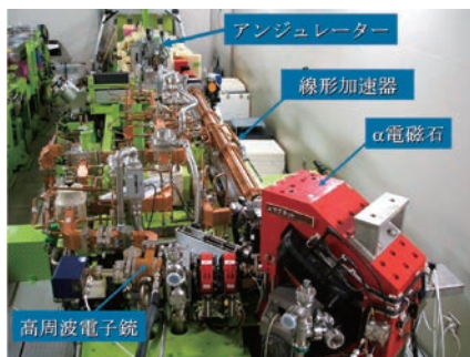
図1 赤外自由電子レーザー本体
