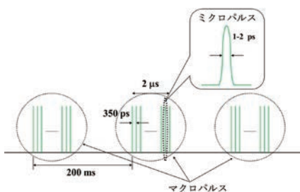
図3 赤外自由電子レーザーのパルス構造
