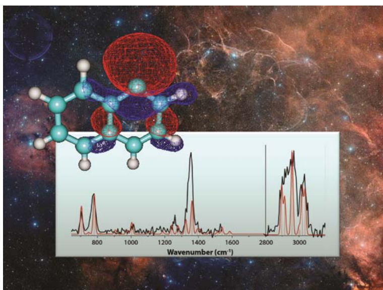
上図は naphthyl 負イオンの赤外スペクトル（黒：実験、赤：理論）
